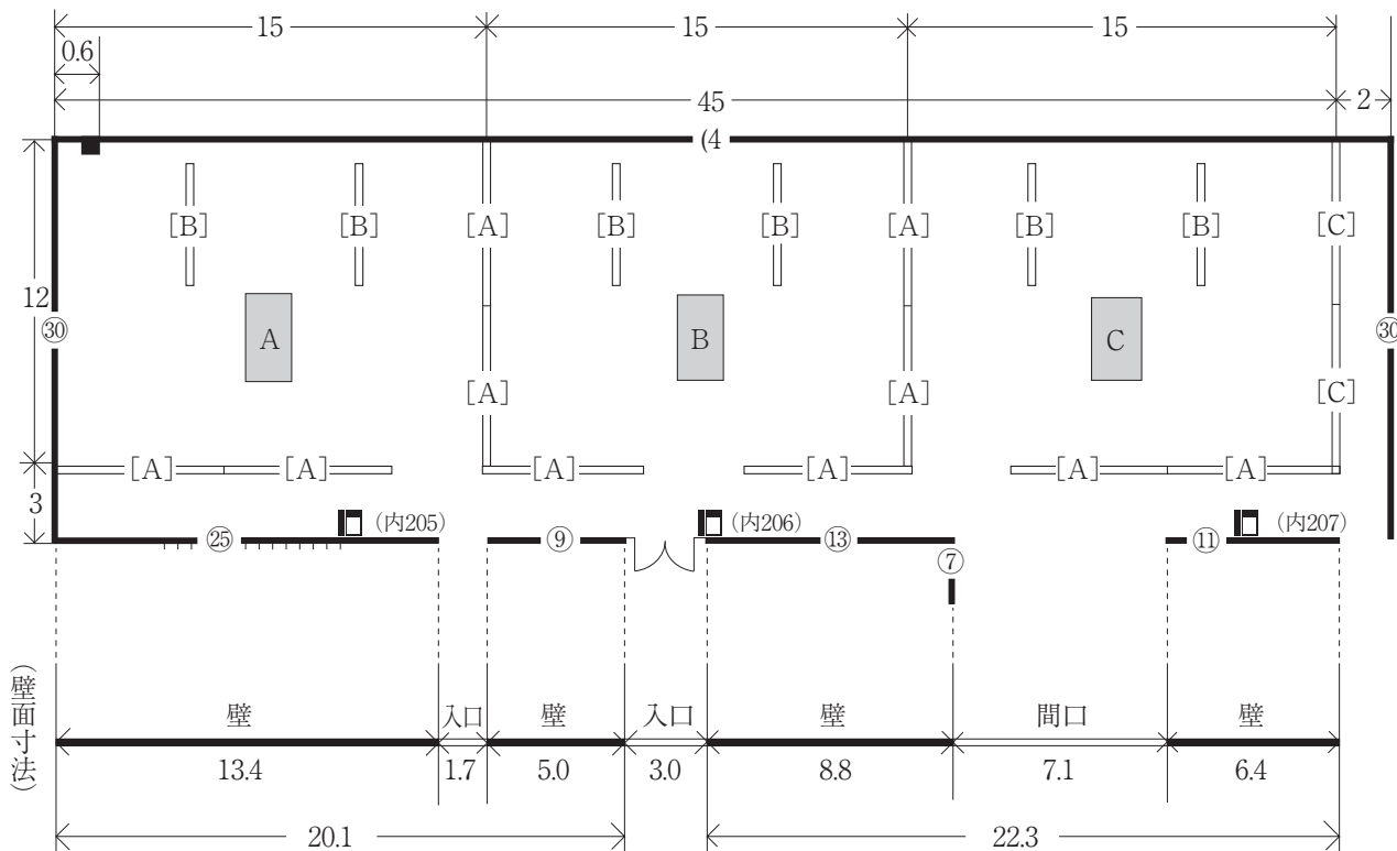
パネルレール図 (レールの無い場所へは移動できません)
