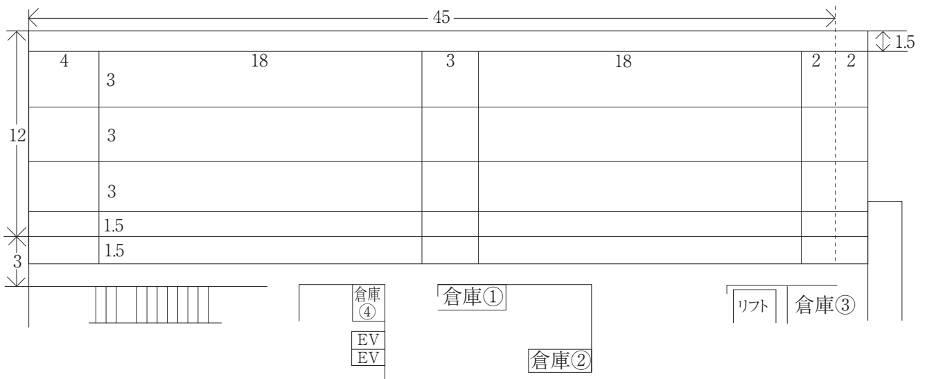
パネルレール図 (レールの無い場所へは移動できません)
